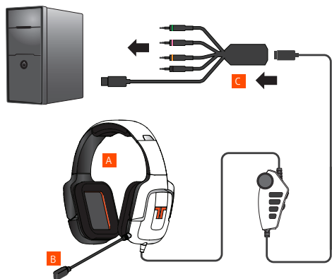
PC - アナログオーディオ接続図
