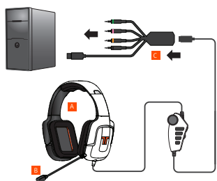
PC - アナログオーディオ接続図
